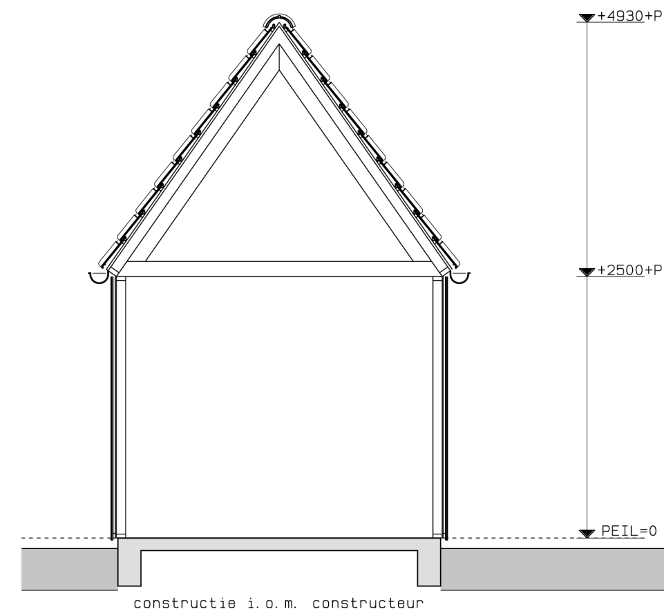
doorsnede
